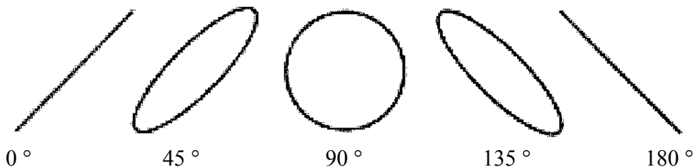
Obr. 10b: Různé úhly fázového posuvu (Lissajousovy obrazce)
